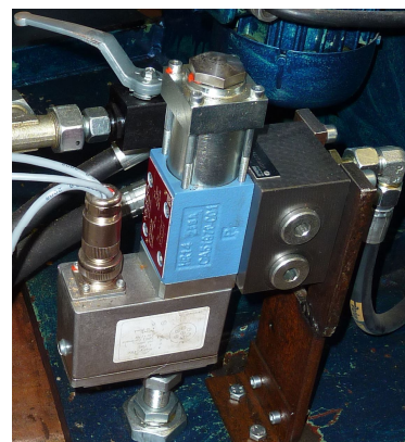
Zawór proporcjonalny
